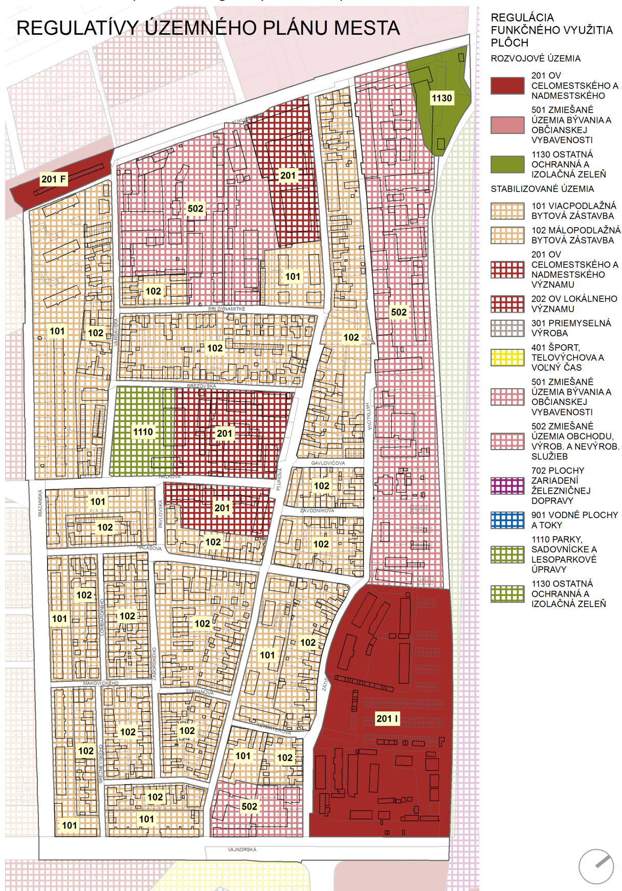
Schéma 3 Funkčné a priestorové regulatívy Územného plánu mesta v riešenom území
