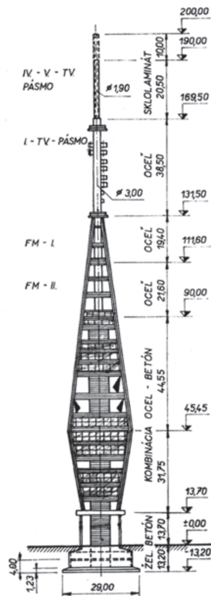
Tvar a konštrukčné materiály veže
